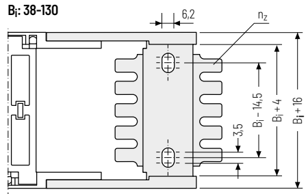
▲ Montagemöglichkeiten
