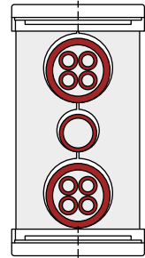
Alloggio ottimale di conduttori in un traversino forato
