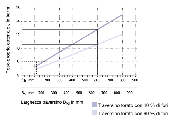
Peso proprio della catena in funzione della larghezza del traversino B_{ST}
