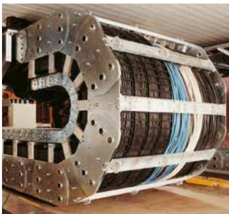
Catene in acciaio con traversini RMA
